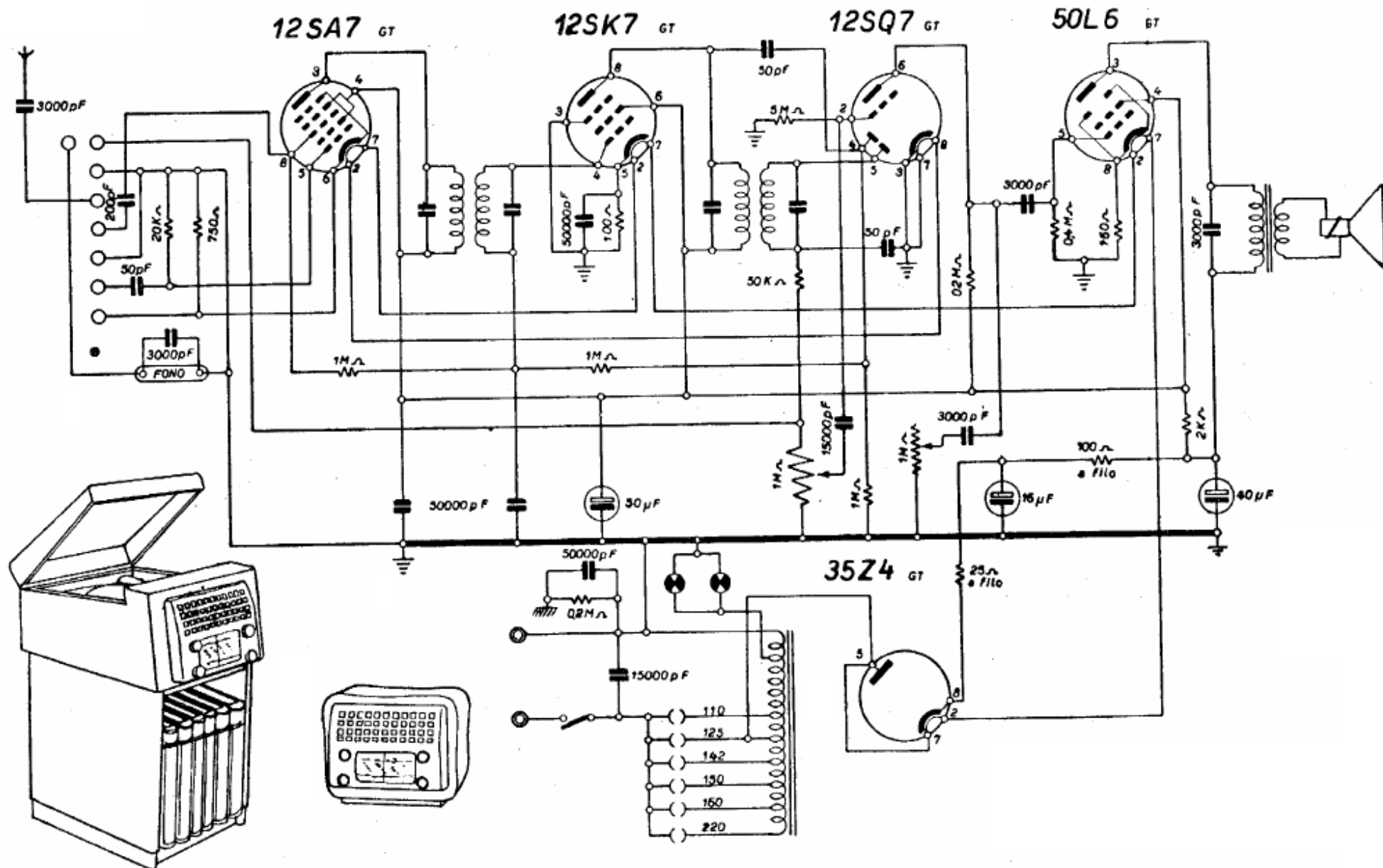
REOM - Sintomagie Radio modelli a1 ed a2 - Il mod. a2 è provvisto di fonografo elettrico. Gamma onde medie divisa e due bande onde corte. Media frequenza 470 kc. Controllo di tonalità.
